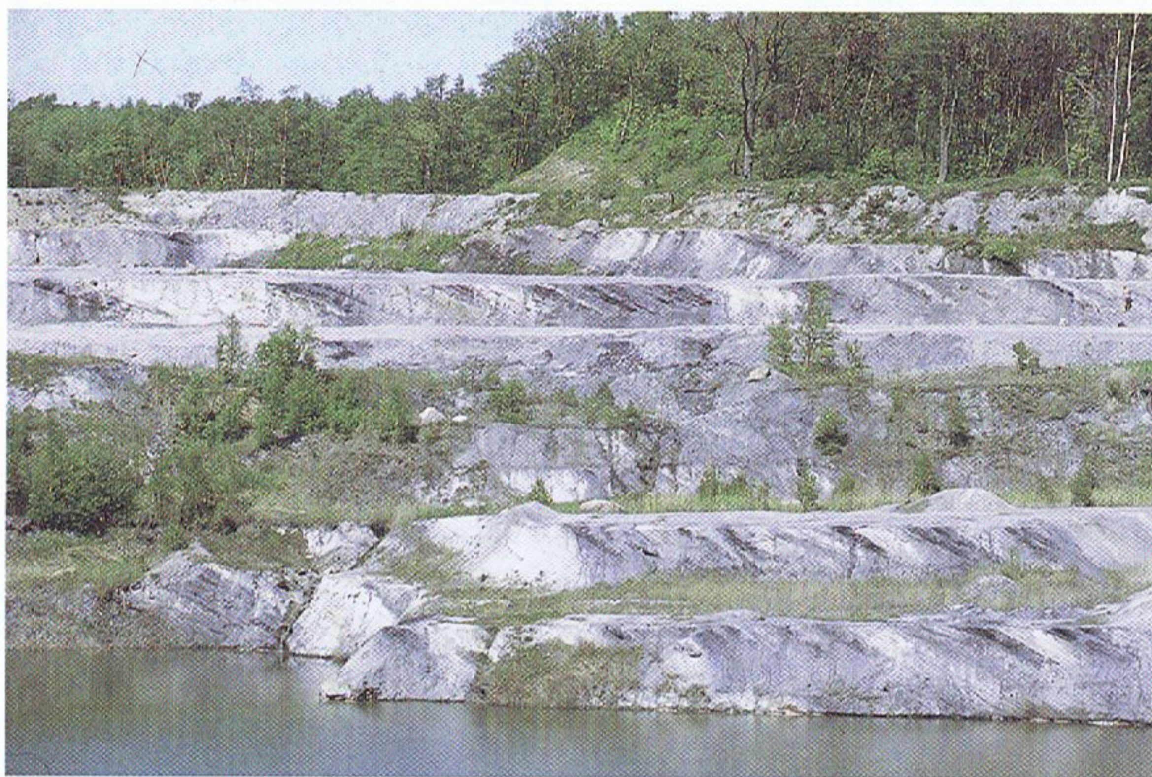
Figur 23. Bagå Formationens vekslende lag af kul, ler og sand fra Mellem Jura. Hasle Klinkerfabriks lergrav. Foto: N. E. Hamann.
