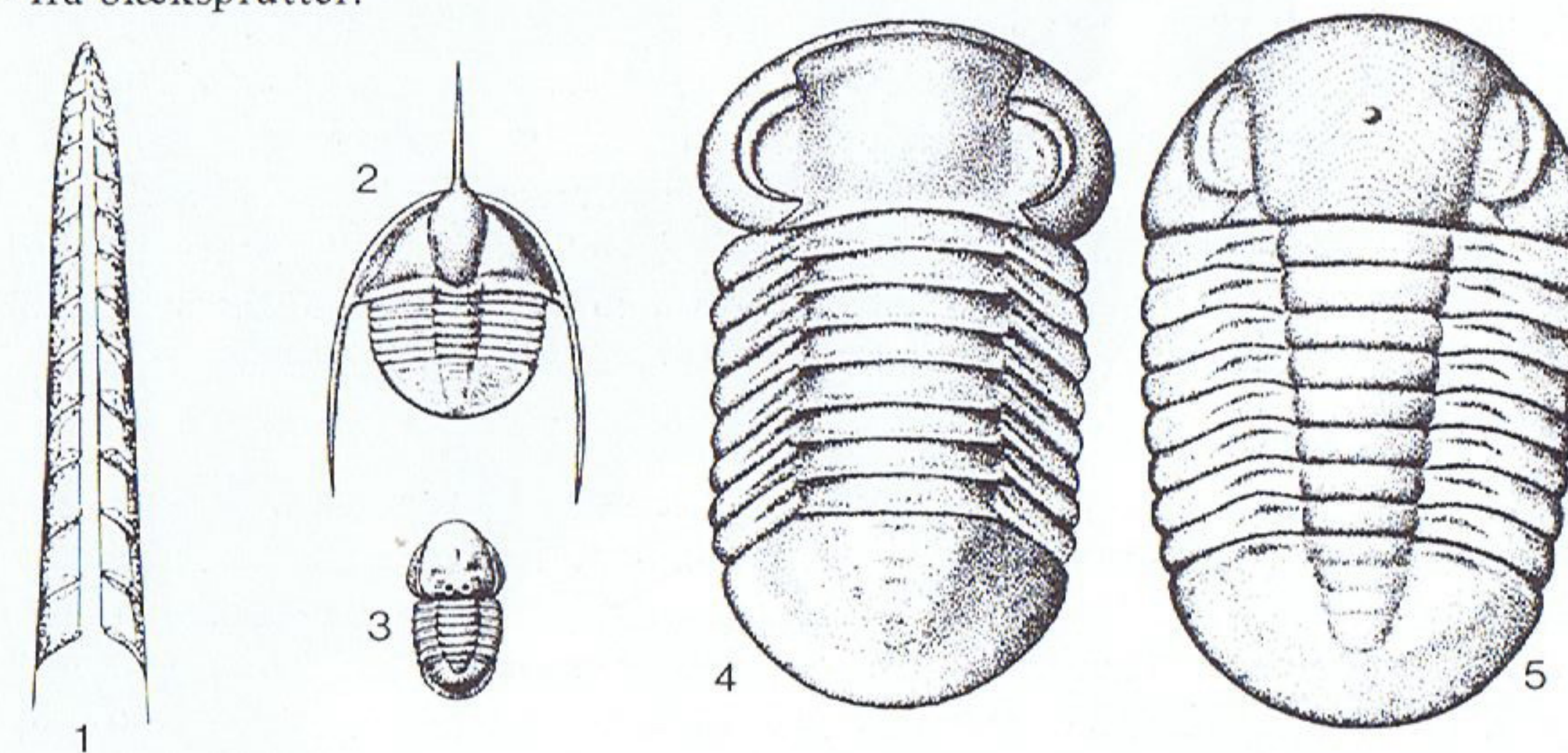
Figur 11. Forstener fra Komstad Kalken (ca. naturlig størrelse). 1. ' Orthoceratit ', Endoceras, 2. Ampyx, 3. Cyclopyge, 4. Nileus og 5. Symphysurus.
