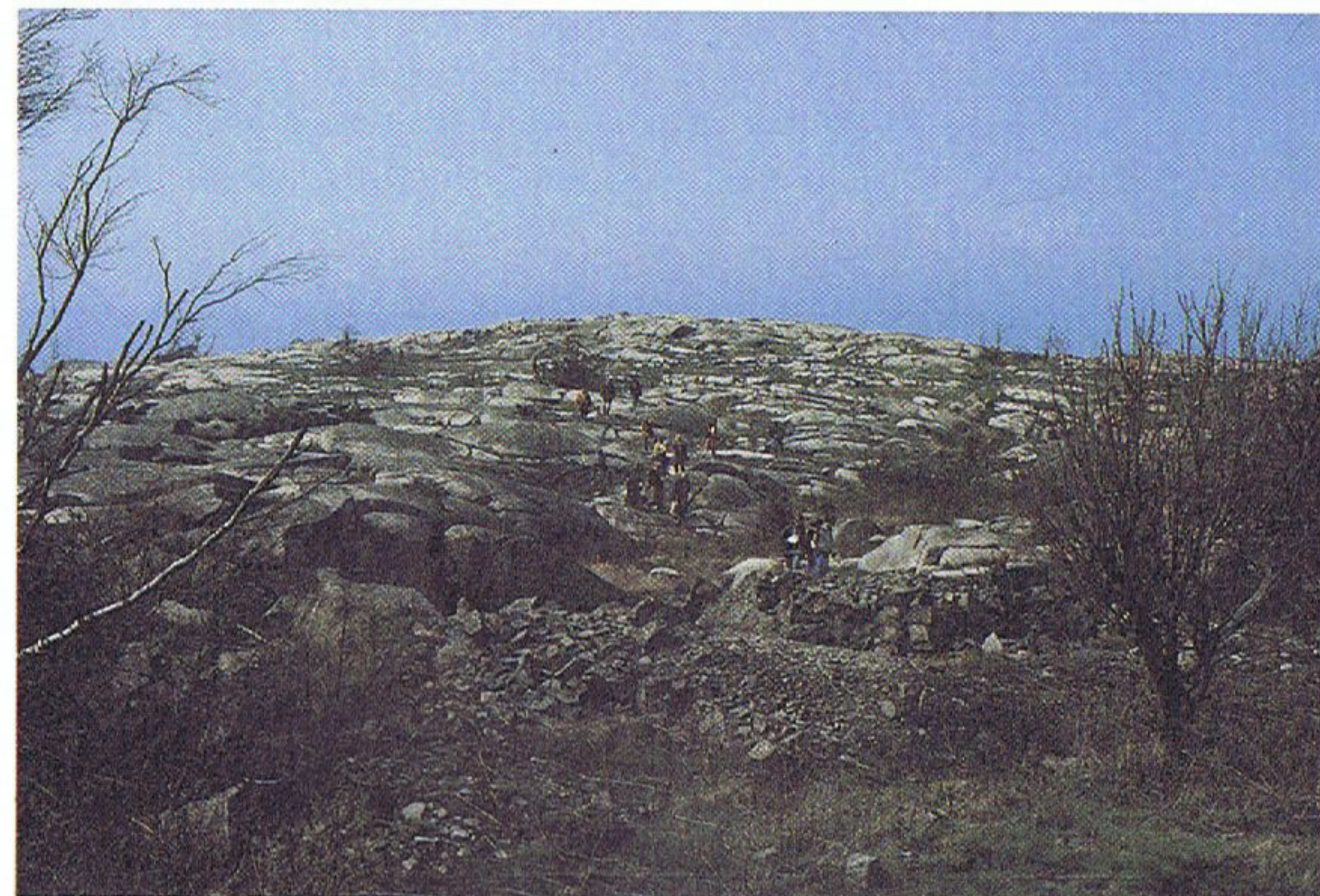
Figur 33. Isafsleben klippeoverflade på Hammerknuden, Nordbornholm. Dels er selve 'Knuden' én stor rundklippe, og dels udgøres overfladen på 'Knuden' af utallige mindre rundklipper. Foto: S. Sjørring.
