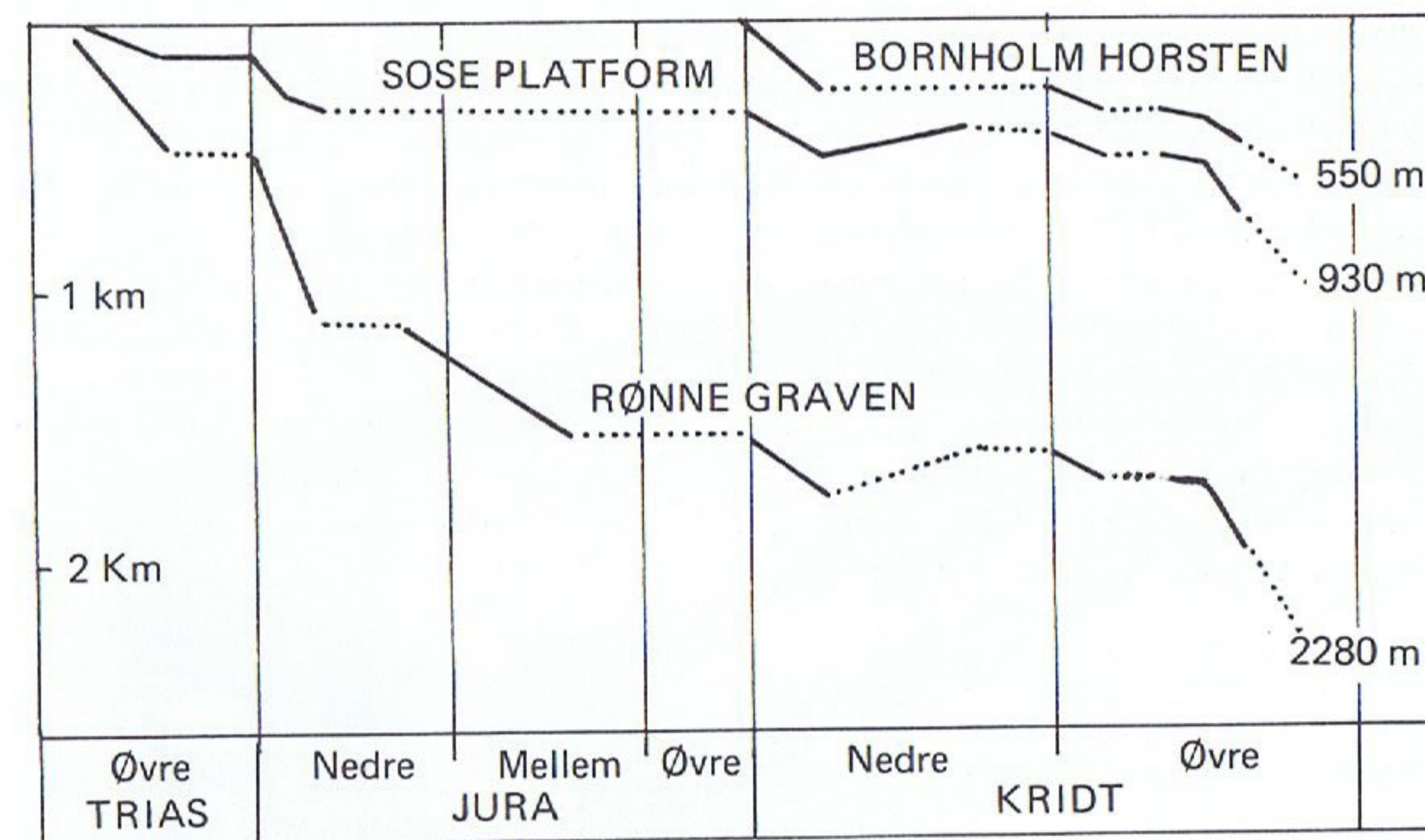
Figur 24. Indsynkningskurver for Bornholm Horsten, Sose Platform og Rønne Gravens østlige del. Kurverne er tegnet på grundlag af aflejringerens nuværende tykkelser, så kurverne 'fortæller' ikke hele sandheden om indsynkningsforholdene. Det ses, at indsynkningen har været nogenlunde ensartet gennem Mesozoikum, men ikke lige hurtigt for de enkelte blokke. Det ses også, at der først afsættes sedimenter på Bornholm Horsten i Kridt.
