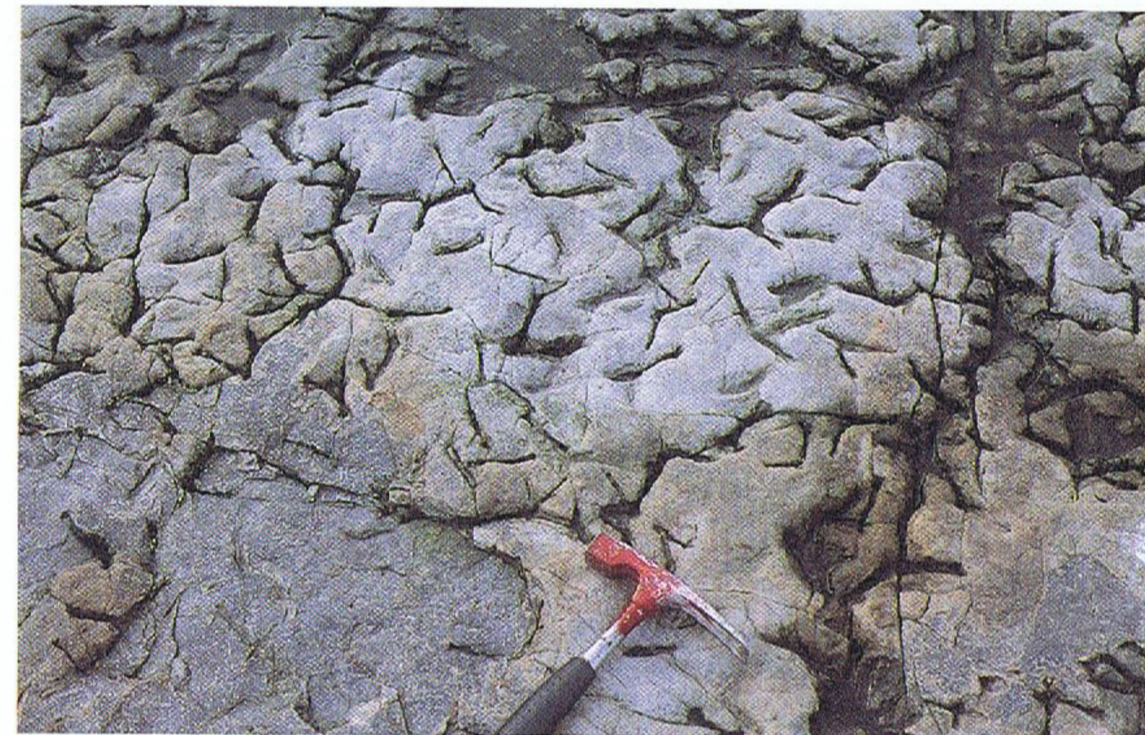
Figur 5. Lagflade med U-formede gravegange (Diplocraterion) lidt nord for Snogebæk havn. Fladen viser et snit igennem de mellemste og nedre dele af gravegangene. På ikke-eroderede flader ses udmundingerne som 'parrede' huller. Foto: S. Sjørring.
