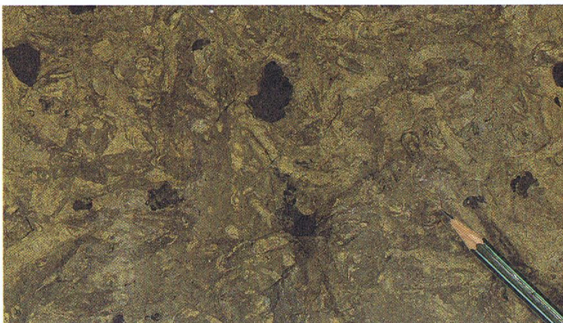
Figur 6. 'Grønne Skifre' med gravegange og sorte fosforitknolde. Fosforiten er udfældet som koncretioner i sedimentet i perioder med ingen eller ringe sedimentation. Ofte er udfældningen sket omkring organisk materiale. Imprægnering med fosforit eller tynde konglomerater med fosforit-rullesten ses mange steder i den Palæozoiske lagsøjle og markerer ophold i sedimentationen. Foto: Ole Bang Berthelsen.
