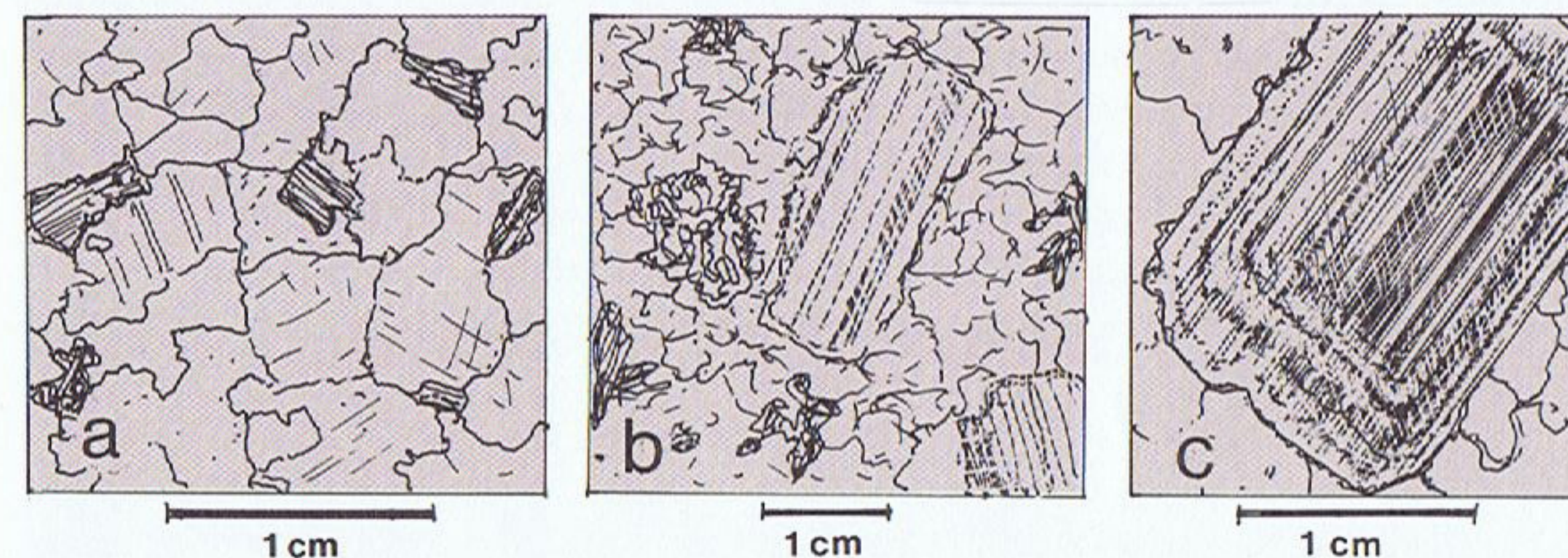
Figur 6. a. Enskornet granit, hvor kornene er vokset 'ligeværdigt', og korngrænserne er uregelmæssige. b. Porfyriske plagioklaskorn med tilnærmet krystalform ses centralt og nederst til højre. Deres vækst var begyndt, før de omgivende mindre korn dannedes. c. Et porfyrisk plagioklaskorn er her zonart udviklet. Plagioklasens calcium-indhold aftager trinvist, og dens natrium-indhold tiltager tilsvarende fra kernen mod randen. Den zonare opbygning afspejler tid- og trinvis ændringer i vækstmiljøet under bjergartens størkning og eventuelle senere omdannelse.
