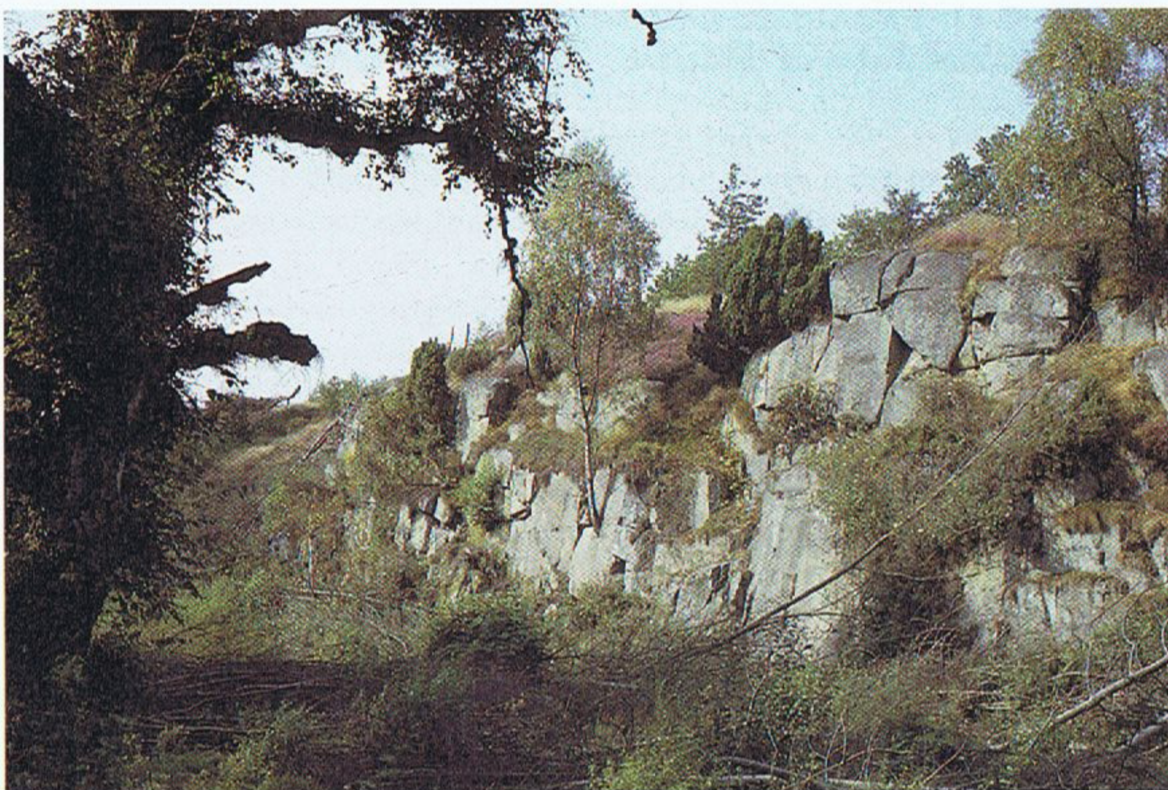
Figur 27. Kodalen: en sprækkedal, hvor indlandsisen har fjernet en stærkt opsprækket diabasgang.
