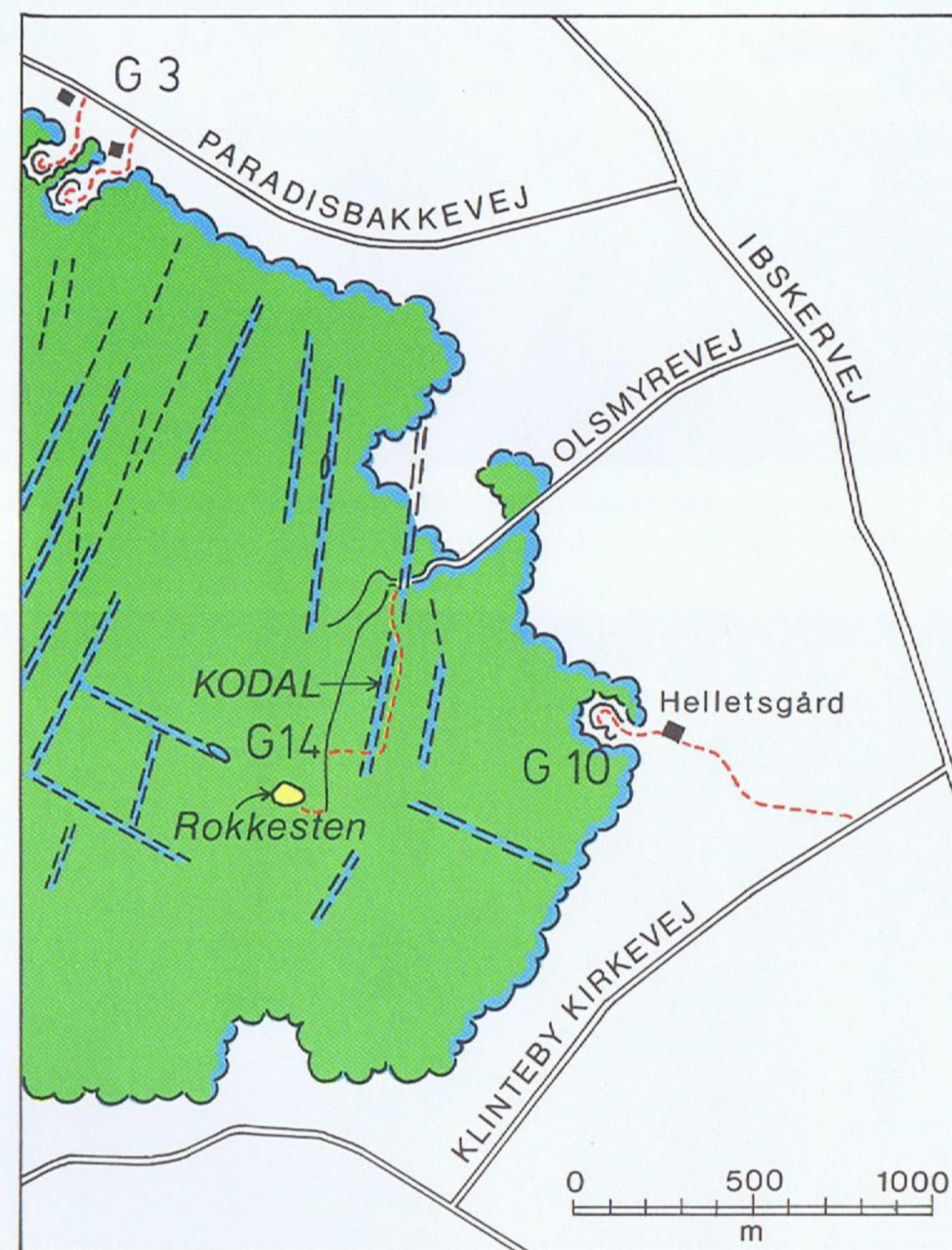
Figur 26. Kortskitse med beliggenheden af lokaliteterne 3, 10 og 14. Større sprækkedal er vist med blå. For enden af Olsmyrevej er der en offentlig parkeringsplads.
