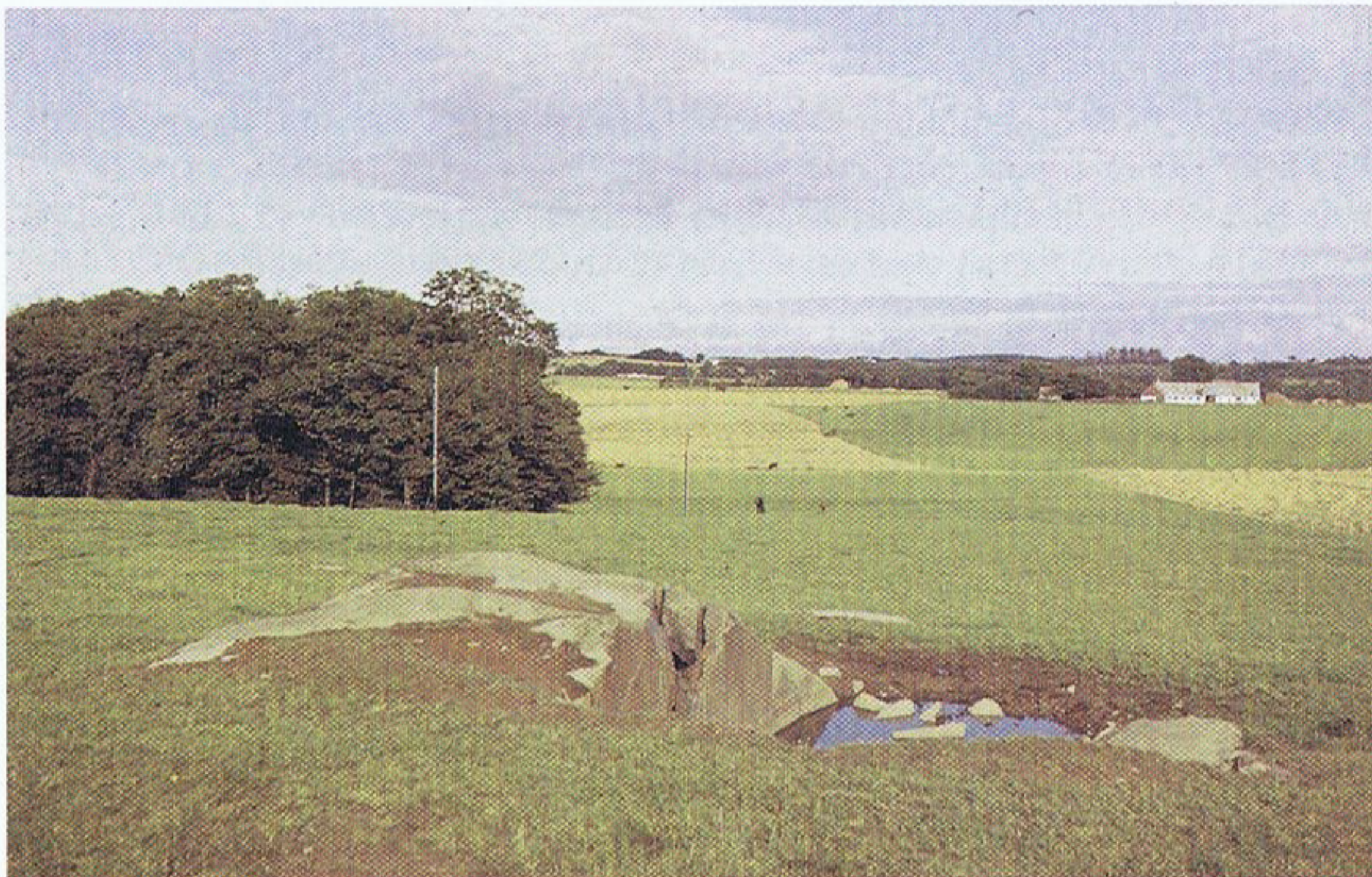
Figur 12. Pyroxen-graniten i markblotning ved Maegård. H. Micheelsen fot.
